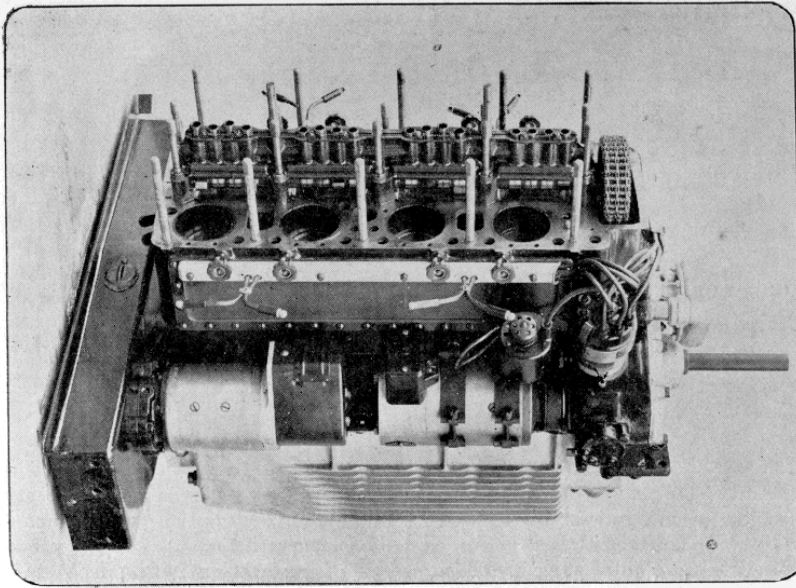
Fig. 3. — Moteur Dilambda, culasse enlevée.
