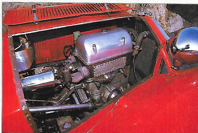
Le V4 à arbre à cames en tête est passé de 2 120 cm 3 au début de sa carrière à 2 570 cm 3 à la fin, et de 49 à 69 chevaux. Le régime maxi de ce moteur, fixé à 3 250 t/mn, était très élevé pour l'époque. La boîte de vitesses ne faisait pas corps avec le bloc, mais était boulonnée sur une traverse derrière le volant d'inertie.
